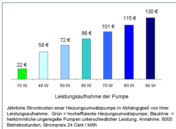
Abb. 2: Vergleich der jährlichen Stromkosten von hocheffizienten Heizungsumwälzpumpen und herkömmlichen Pumpen mit unterschiedlicher Leistungsaufnahme.
