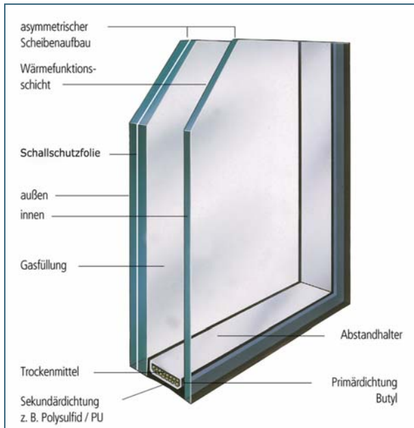
Abb. 5: Schematischer Aufbau einer 2-Scheiben-Schallschutzverglasung
