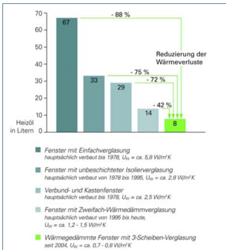
Abb. 2: Jährlicher Wärmeverlust pro Quadratmeter Fensterfläche unterschiedlicher Fenstertypen umgerechnet in Liter Heizöl
